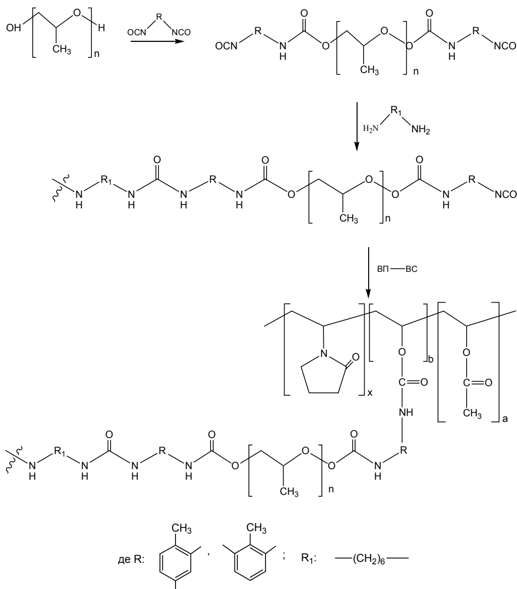
Рис. 1. Схема реакції синтезу ПУС, які містять у своїй структурі фрагменти кополімеру ВП–ВС
