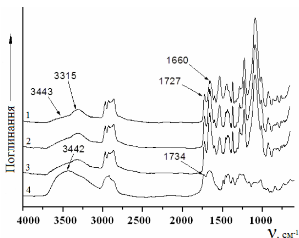
Рис. 3. ІЧ-спектри синтезованих ПУС:
