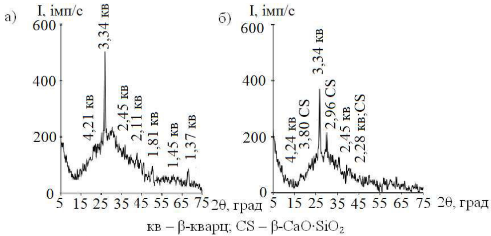
Рентгенограми дослідних зразків з різною тривалістю ізотермічного витримання: а – 10 хв; б – 60 хв
